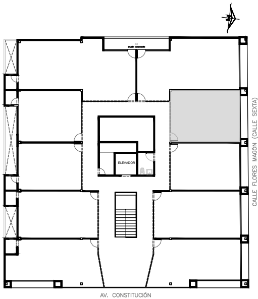
UBICACIÓN EN ELEVACIÓN ARQUITECTÓNICA, NIVEL 4
